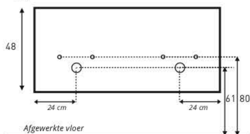
Achteraanzicht tbv aan- /afvoer UFO met frame DUBBEL 120
